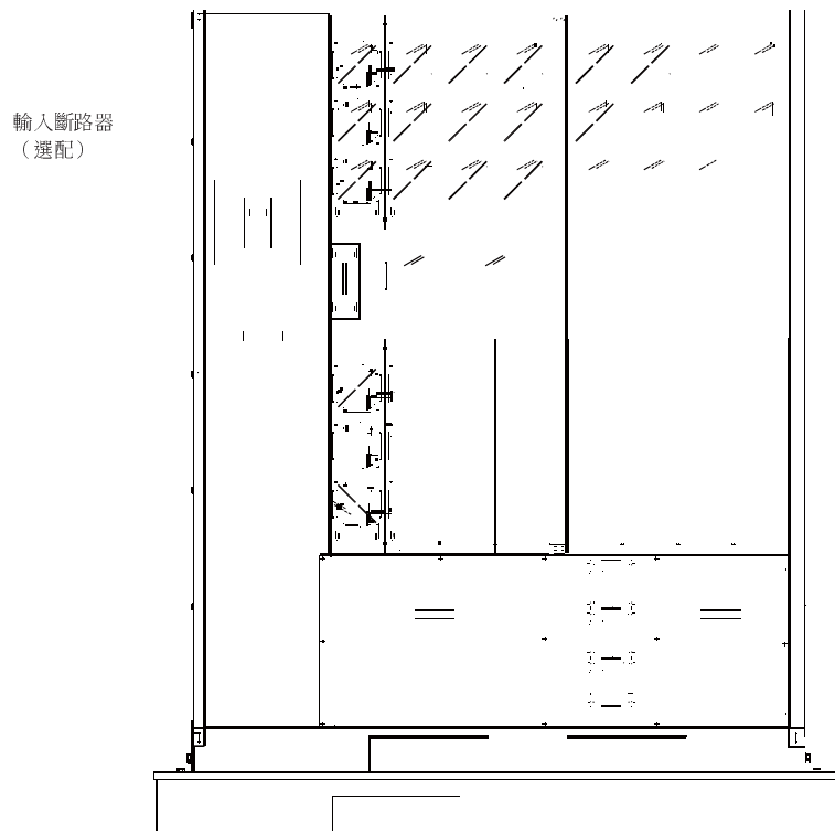
圖 6-2 : UPS 斷路器
