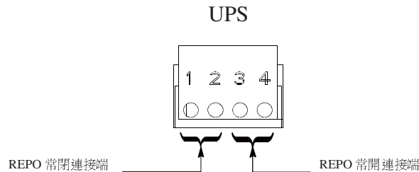
圖 4-7. REPO 端子排介面線分配
