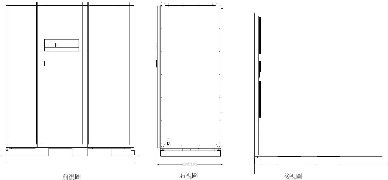
圖 3-2：UPS 機櫃尺寸 (前視圖、右視圖及後視圖) 單位：毫米 [英寸]
