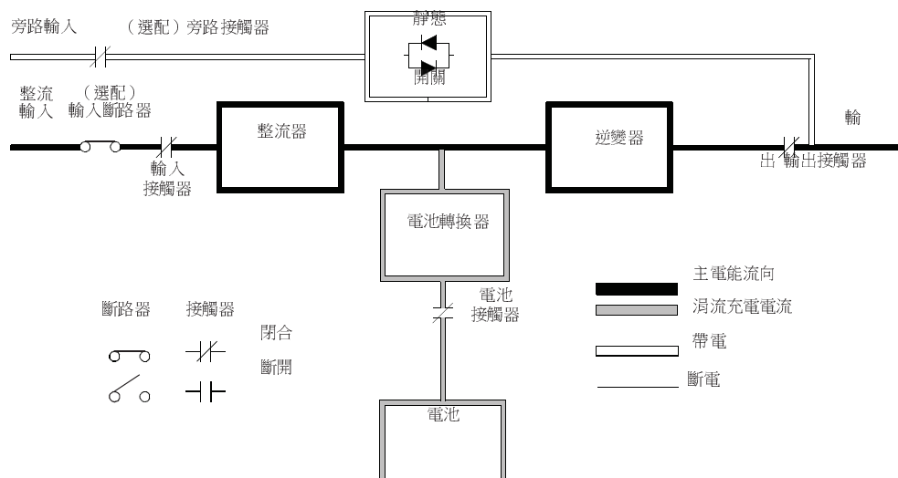
圖 5-2：“標準正常”模式下電能通過 UPS 的路徑
