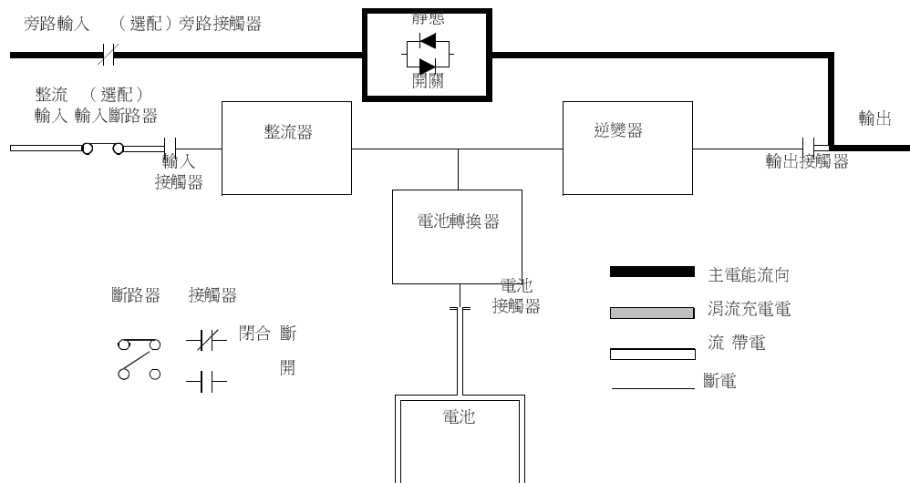
圖 5-3：“旁路”模式下電能通過 UPS 的路徑
