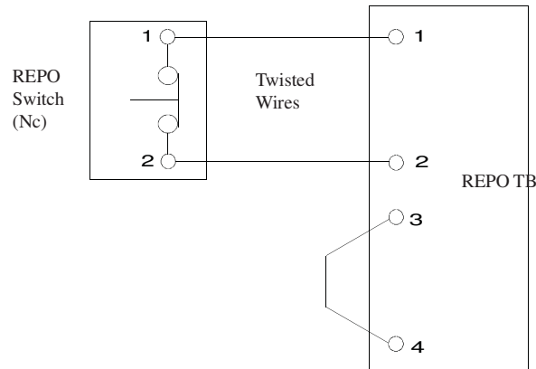
圖 4-9：常閉 REPO 開關配線
