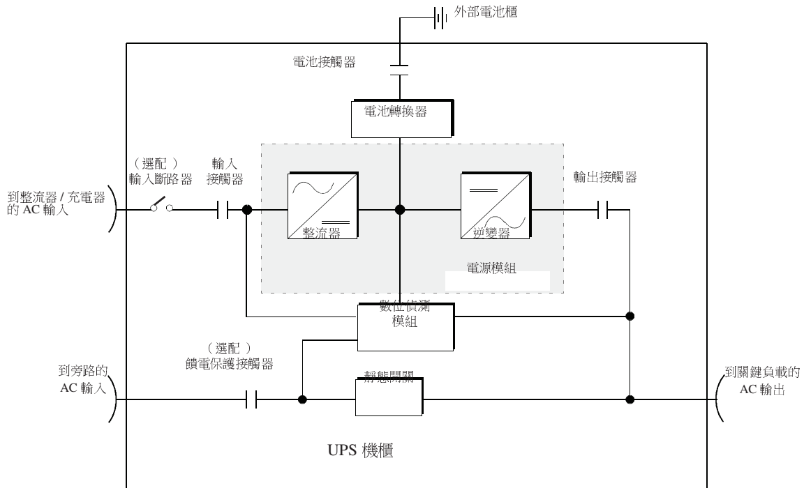
圖 5-1：UPS 系統的主要原理
