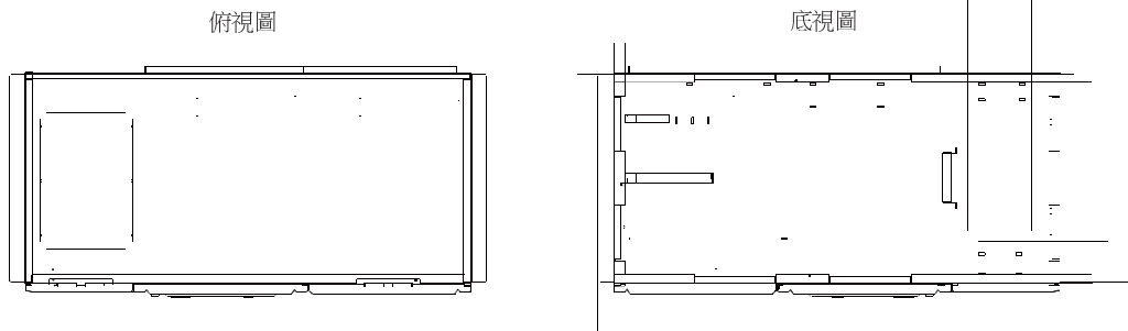
圖 3-1：UPS 機櫃尺寸 (俯視圖及底視圖) 單位：毫米 [英寸]
