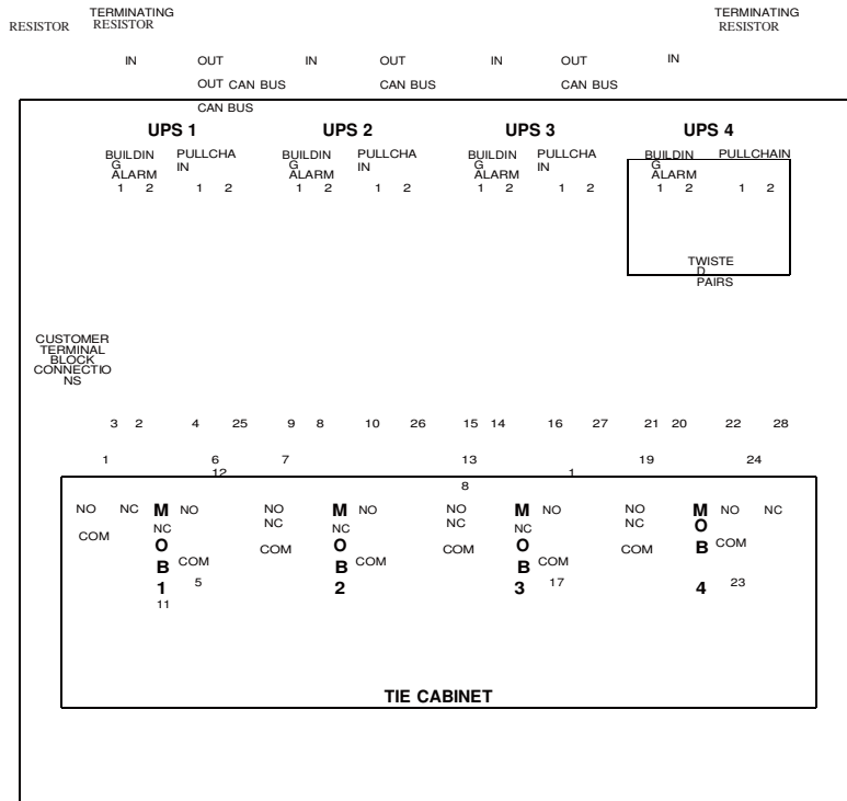
並機信號線和 CAN 通訊控制線接線圖
