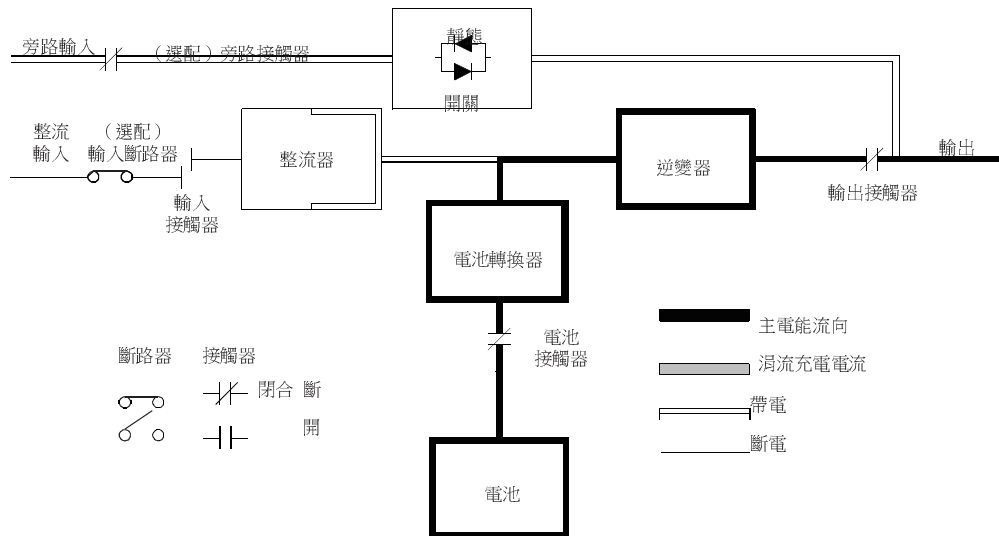
圖 5-4：“電池”模式下電能通過 UPS 的路徑
