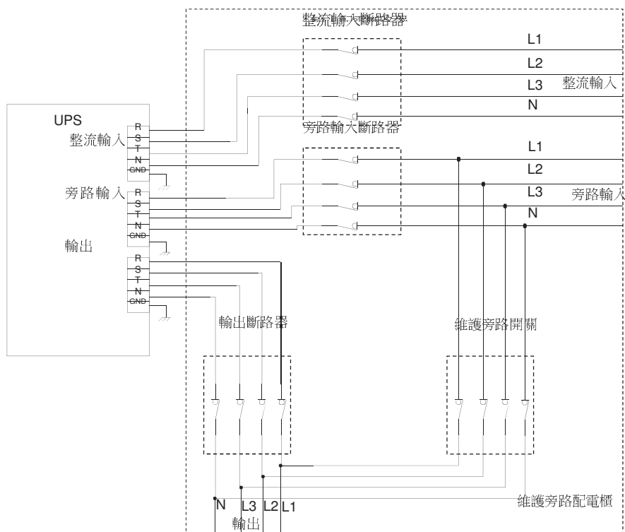
圖 6-8：外部維護旁路安裝示意圖
