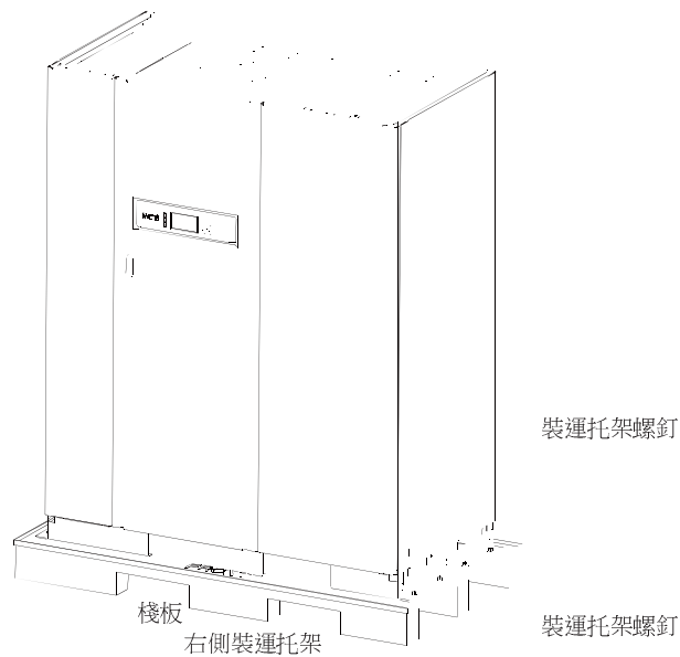
圖 4-1：拆除裝運托架
