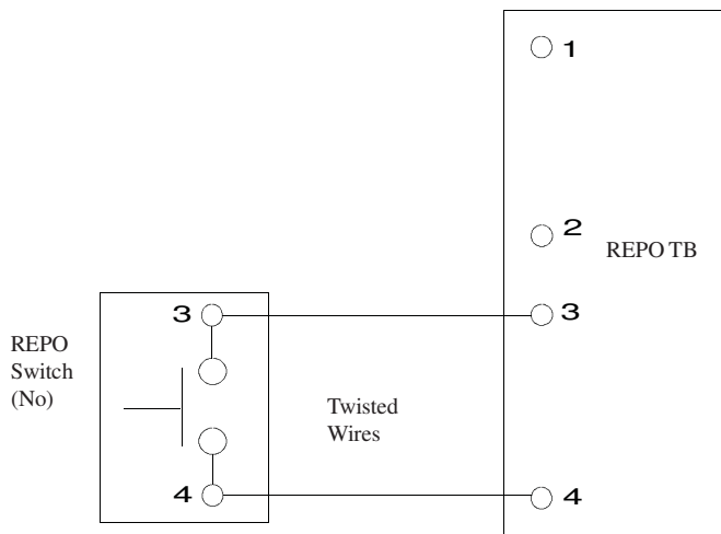
圖 4-8：常開 REPO 開關配線
