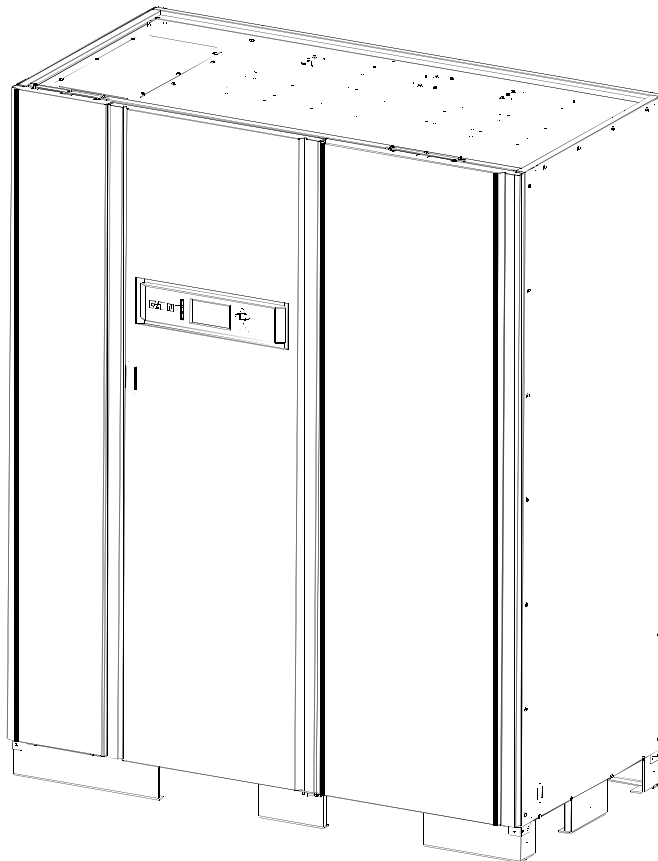
圖 1-1：Eaton 93E 300/400 kVA UPS
