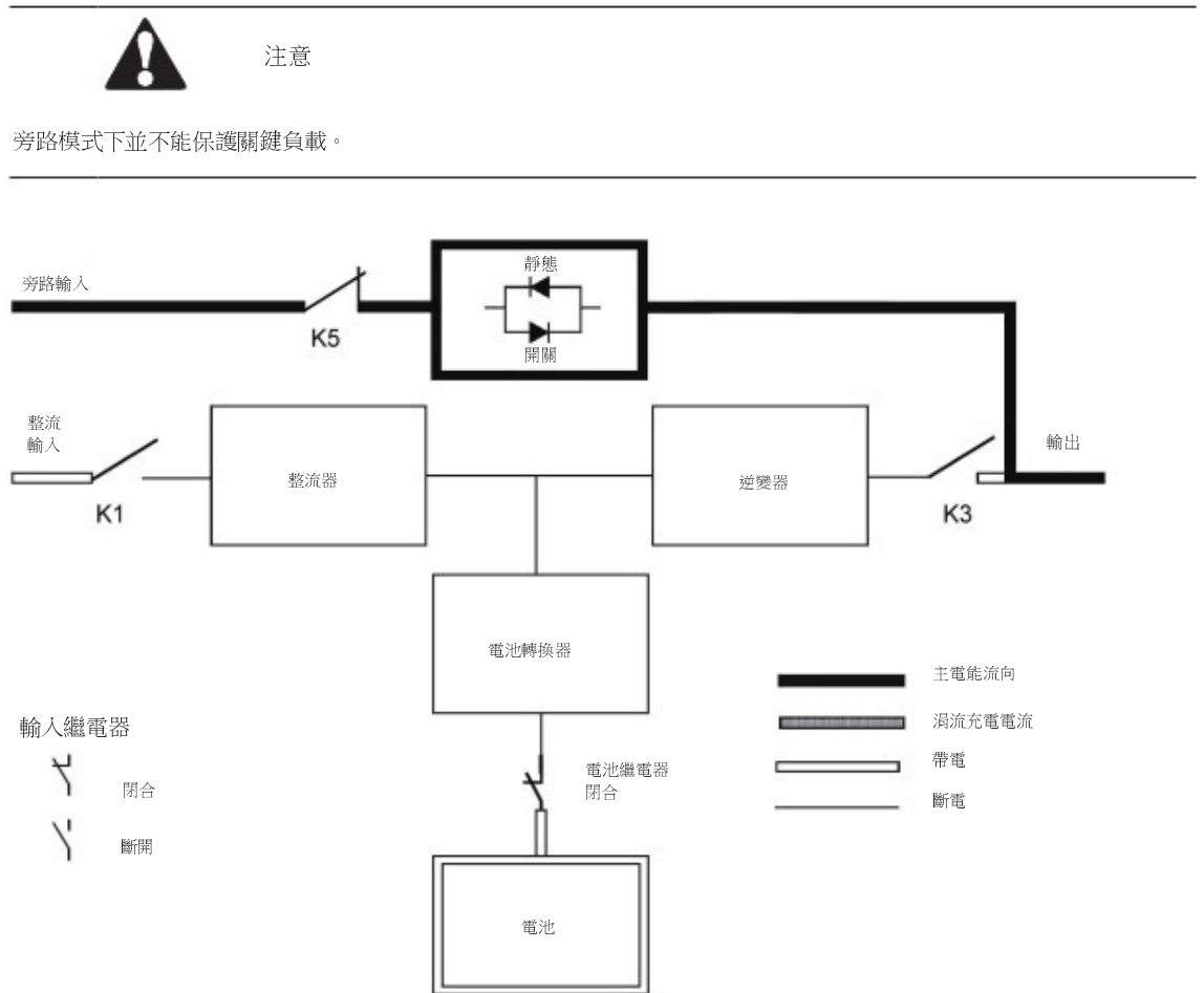
圖 2-7：旁路模式電能通過 UPS 的路徑
