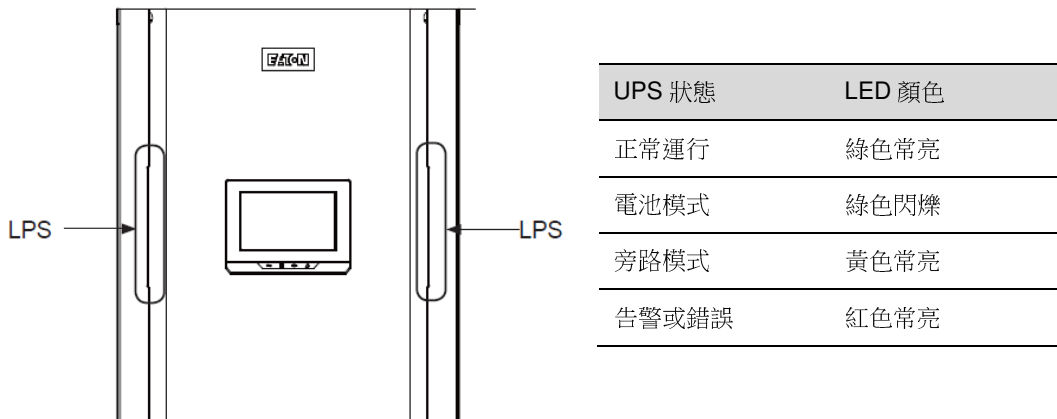
圖 6-7：LED 燈條
