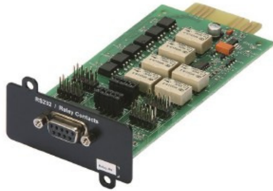
圖 5-4 : Relay Card-MS
