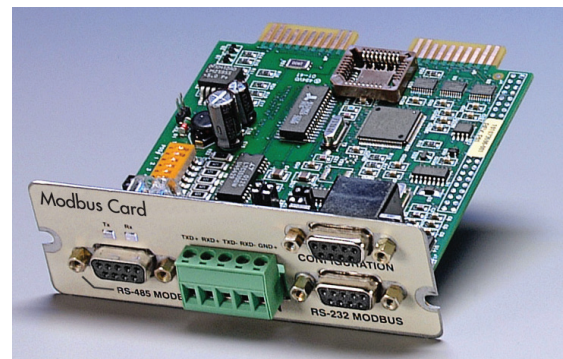
圖二：MODBUS 通訊卡
