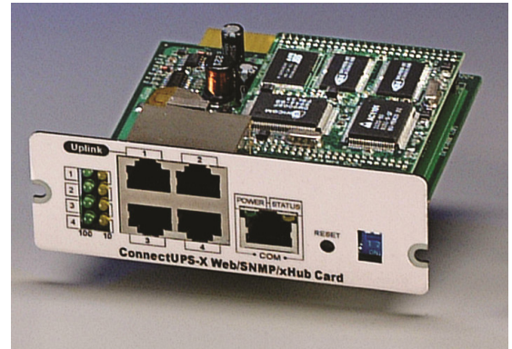
圖一：SNMP/Web Hub卡
