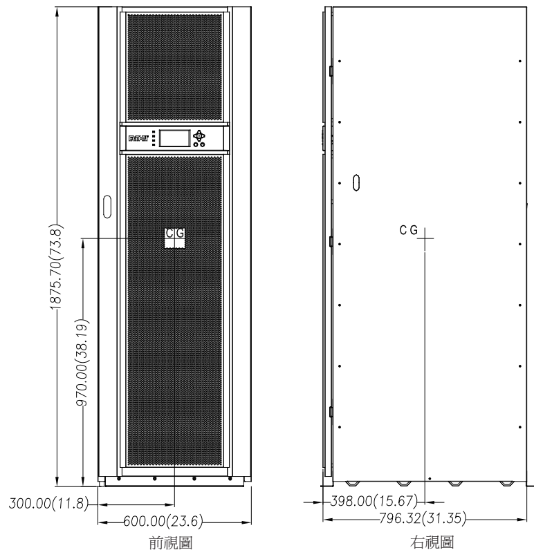
圖 3-3：UPS 機櫃重心
