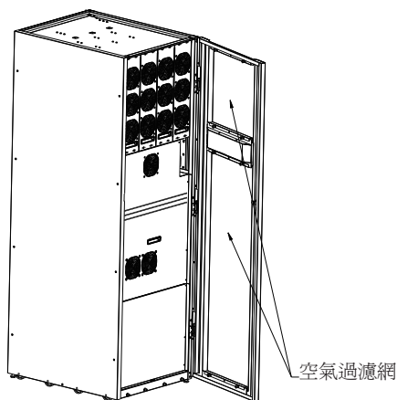
圖 8-1：空氣過濾網位置
