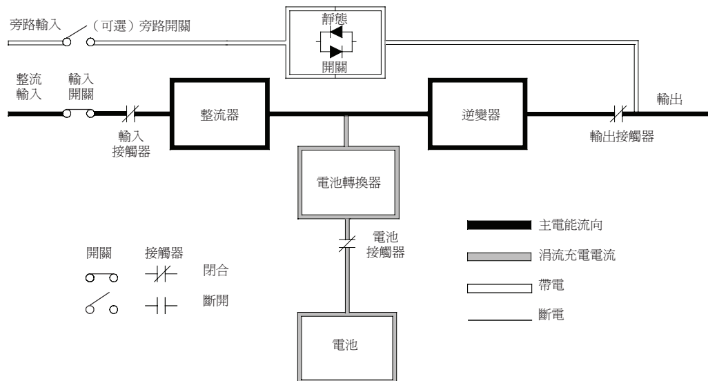
圖 5-2：“標準正常”模式下電能通過 UPS 的路徑
