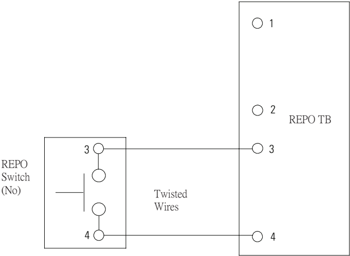
圖 4-17：常開 REPO 開關配線
