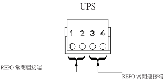
圖4-16. REPO 端子台接點線分配
