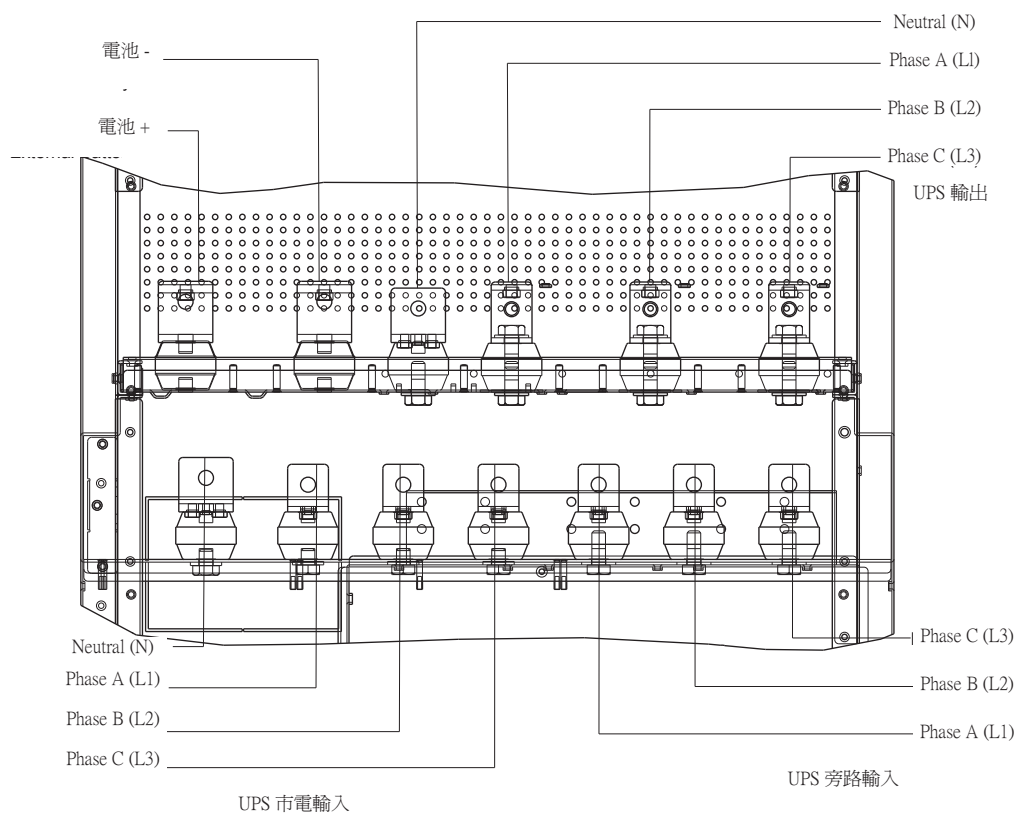
圖 4-7. 電源端子台位置詳圖 160-200 kVA
