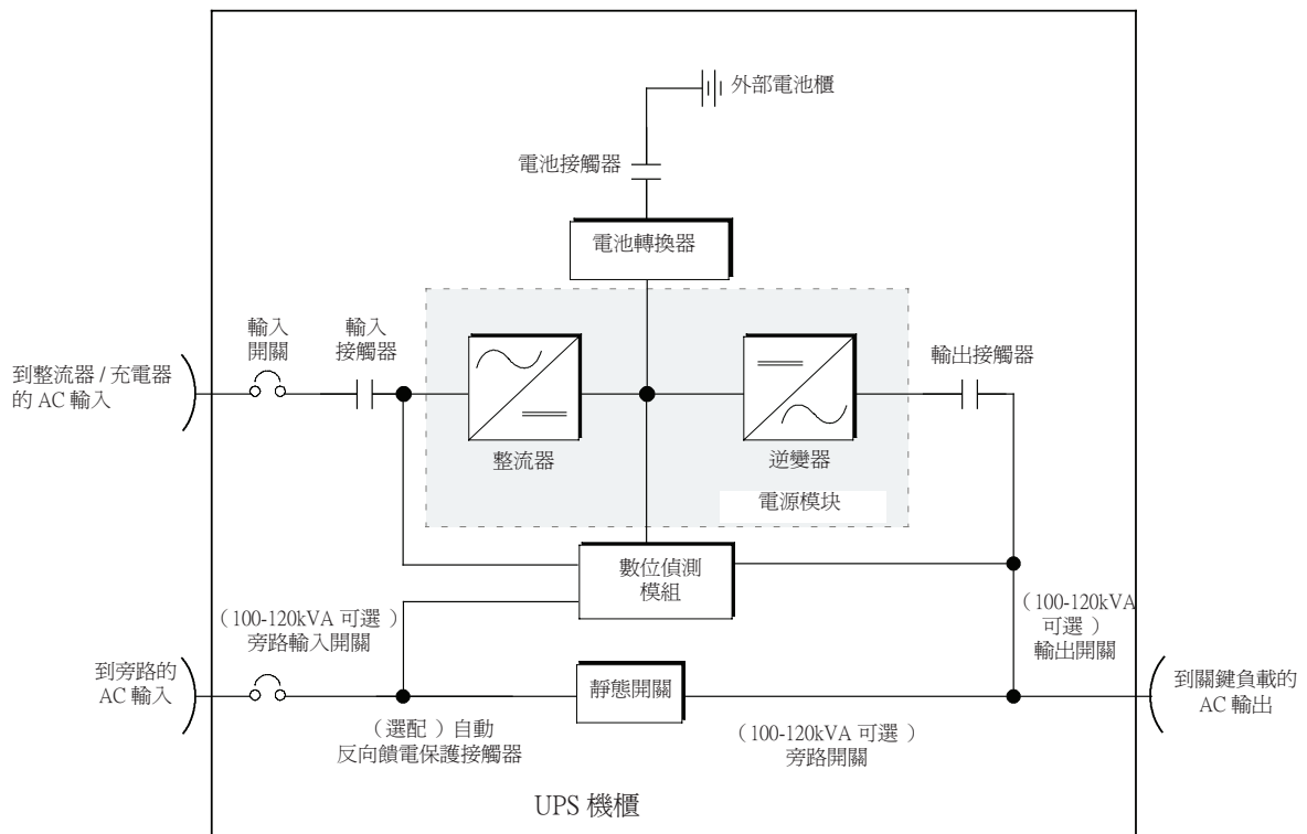
圖 5-1：UPS 系統的主要原理
