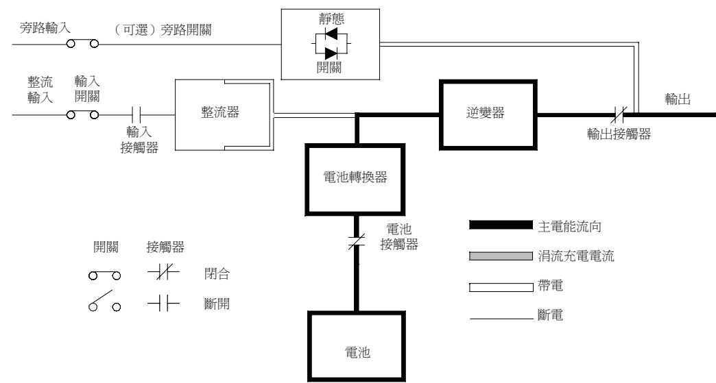
圖 5-4：“電池”模式下電能通過 UPS 的路徑
