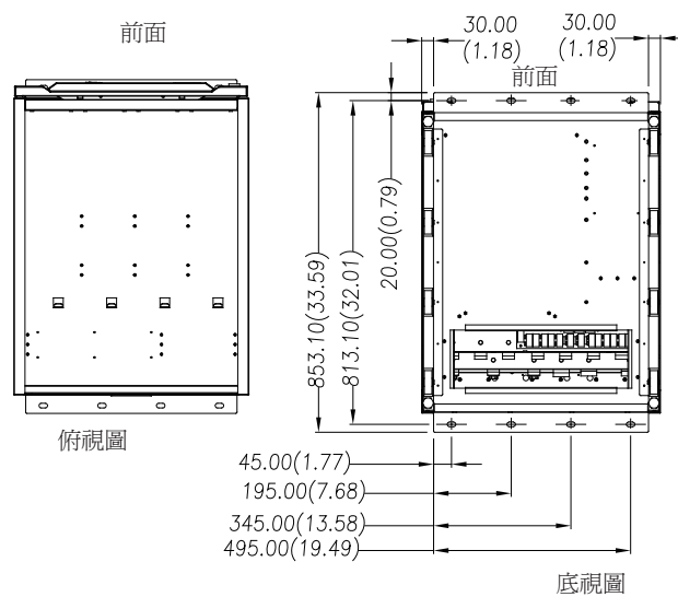
圖 3-2：UPS 機櫃尺寸 (俯視圖及底視圖)
