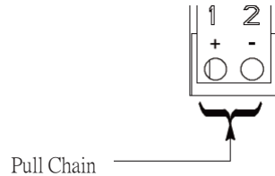
圖 4-13. 並機線端子台接點分配
