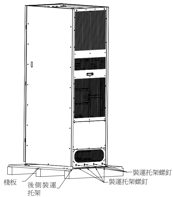
圖 4-3：拆除背面裝運托架
