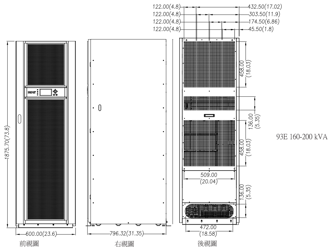
圖 3-1：UPS 機櫃尺寸（前視圖、右視圖及後視圖）
