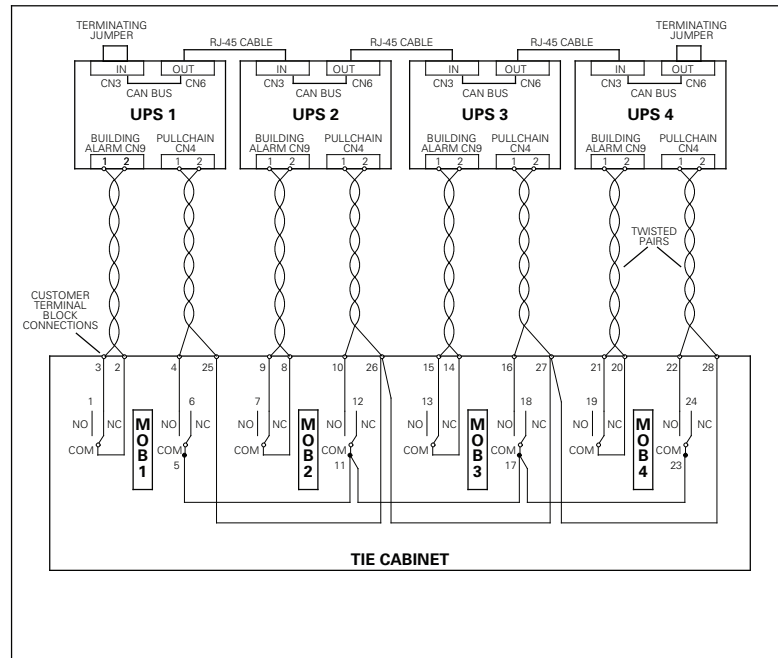
並機信號線與 CNA 通訊控制線接線圖
