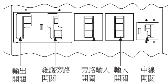
圖6-8：100-120kVA 可選內部維護旁路開關佈置
