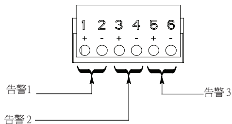
圖4-11. 告警端子台接點分配
