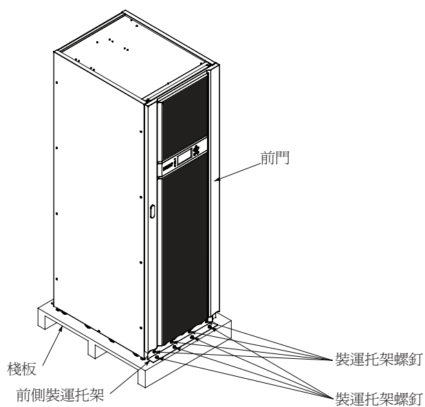
圖 4-1：拆除正面裝運托架
