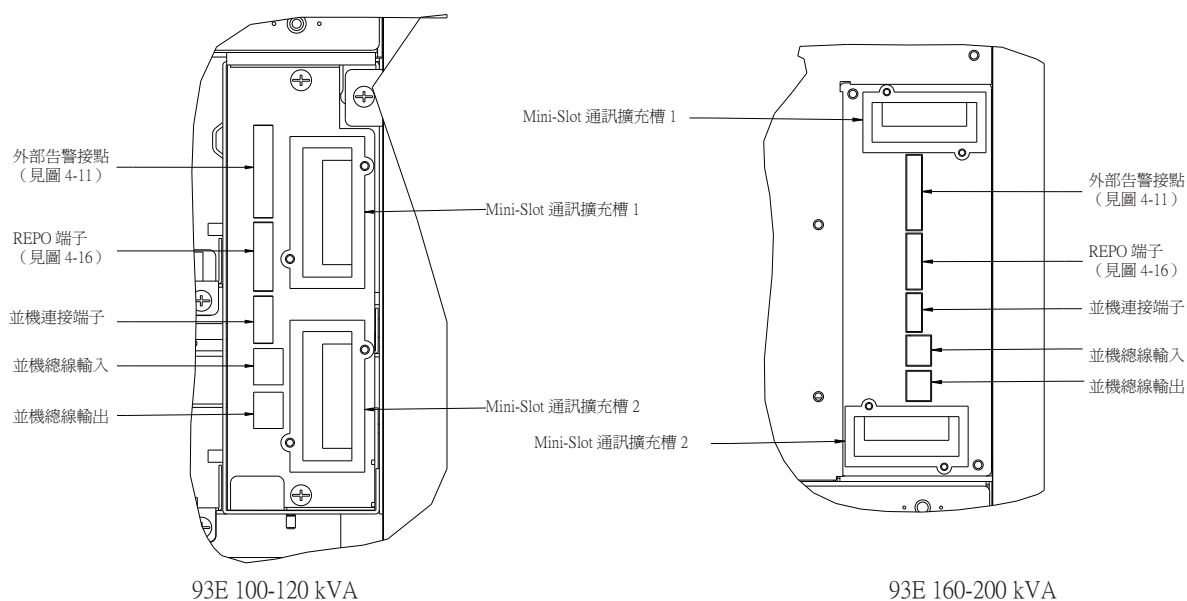
圖4-10. 外部接點端子詳圖
