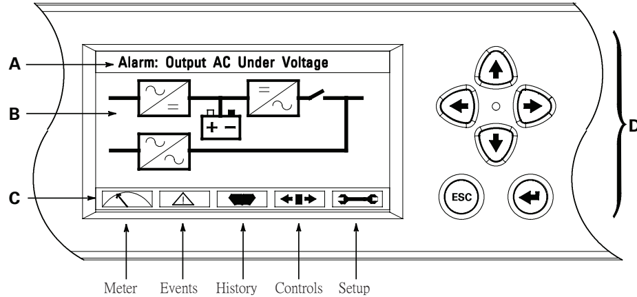
圖 6-4：LCD 的顯示區
