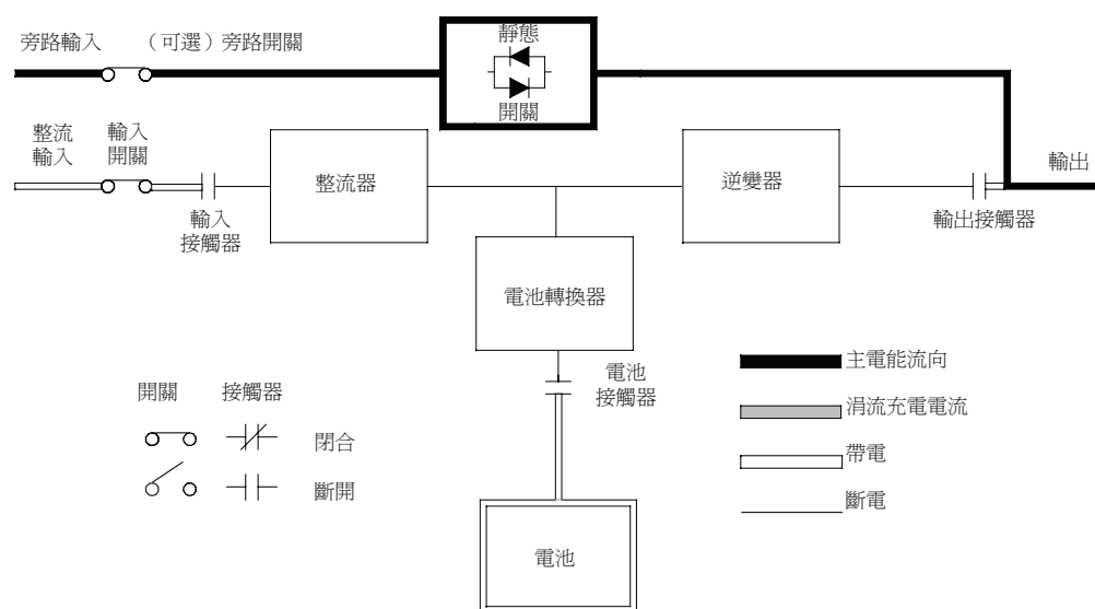
圖 5-3：“旁路”模式下電能通過 UPS 的路徑
