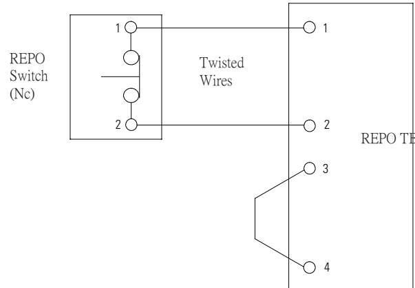
圖 4-18：常閉 REPO 開關配線
