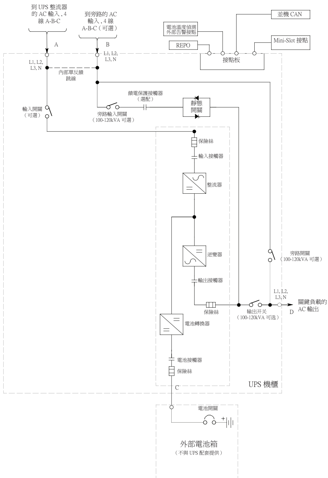
圖 5-5：UPS 系統單線結構 說明：字母 A, B 和 D 對應表 3-5。
