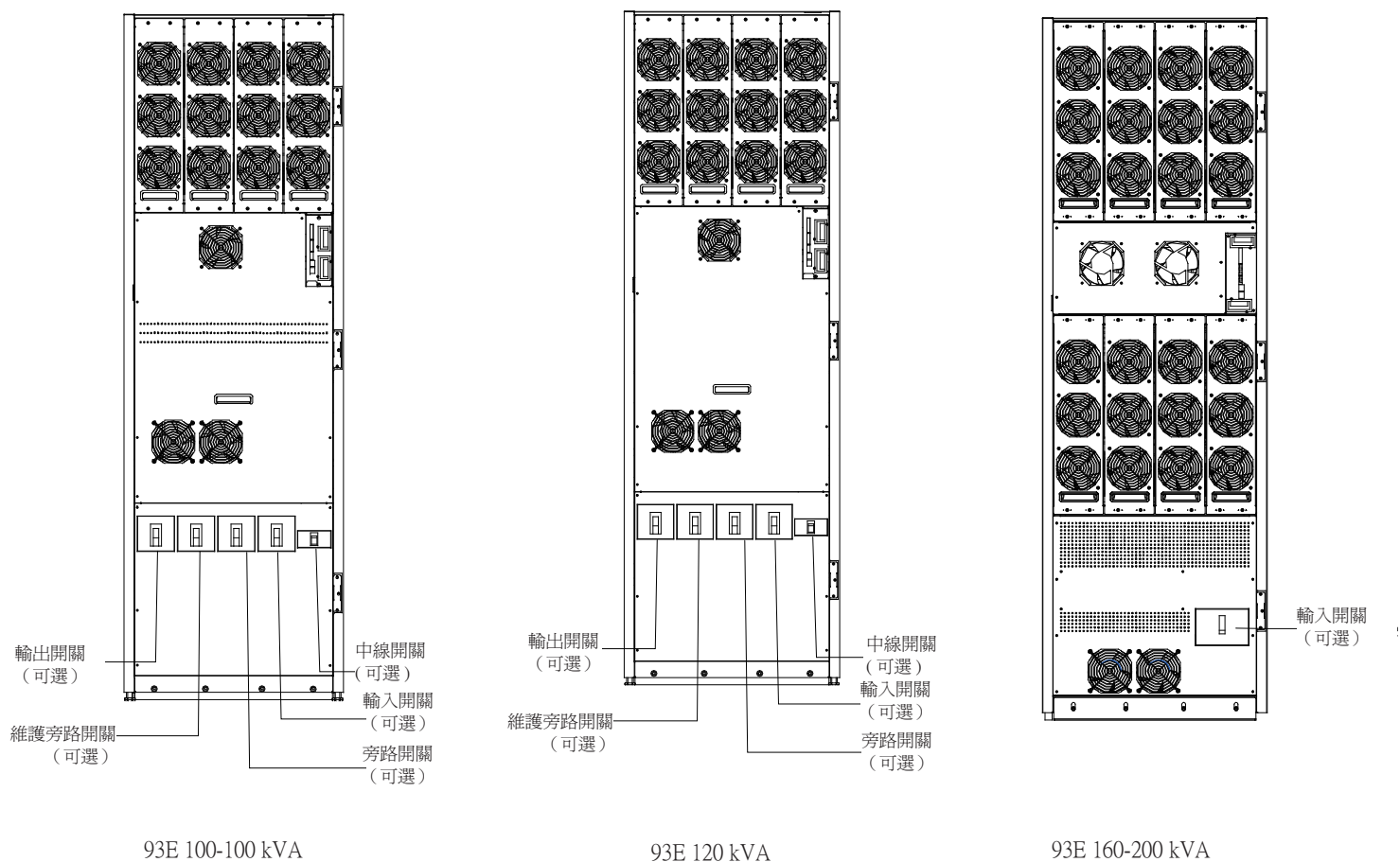
圖 6-2：UPS 斷路開關
